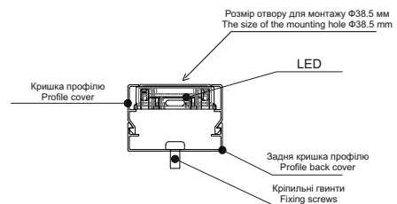
Монтаж профілю: другий спосіб Profile installation: the second method
