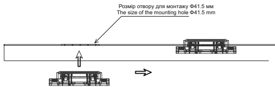
Монтаж профілю: перший спосіб Profile installation: the first method
