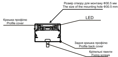
Монтаж профілю: другий спосіб Profile installation: the second method
