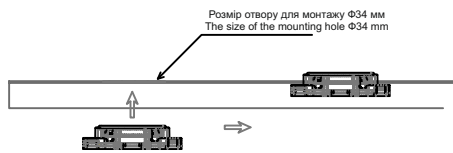
Монтаж профілю: перший спосіб Profile installation: the first method
