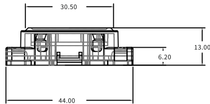
Монтаж профілю: другий спосіб Profile installation: the second method
